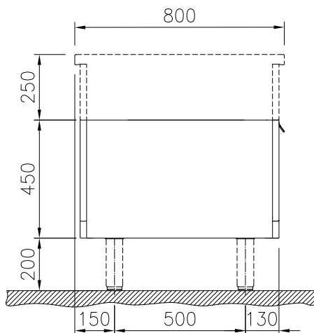
Boven aanzicht
